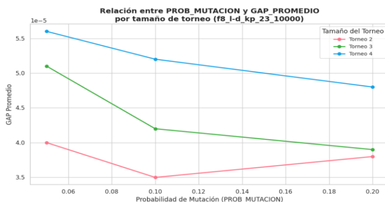
Figura N°15. Variación del GAP promedio en función de la probabilidad de mutación para distintos tamaños de torneo para el dataset f8_l-d_kp_23_10000.txt.
