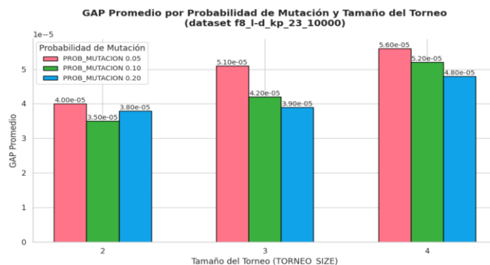
Figura N°16. Comparación del GAP promedio para diferentes tamaños de torneo y probabilidades de mutación para el dataset f8_l-d_kp_23_10000.txt.
